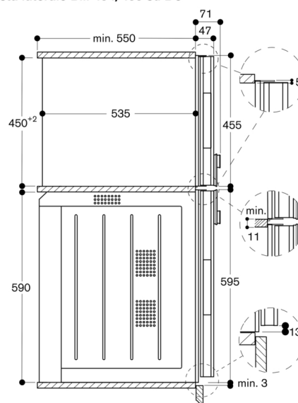
Vista laterale BM 454/455 su BO
