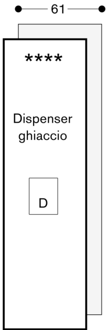
Distanza dalla parete RB 472/RC/RF/RW
