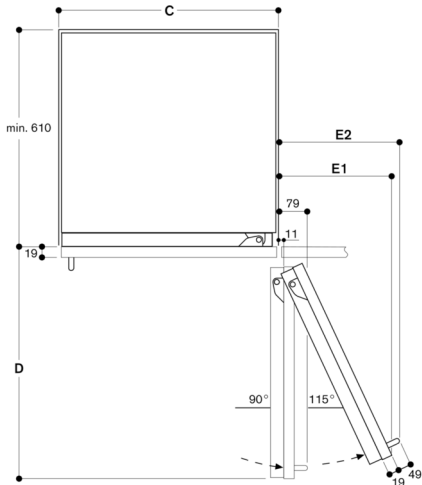
Distanza dalla parete RB 472/RC/RF/RW
