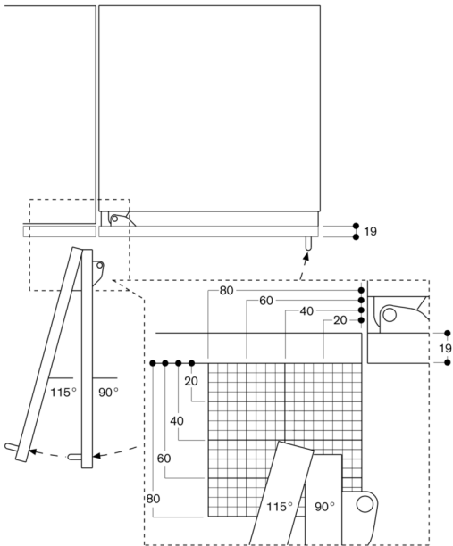
Angolo d'apertura porta
