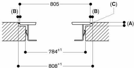
Sezione longitudinale
