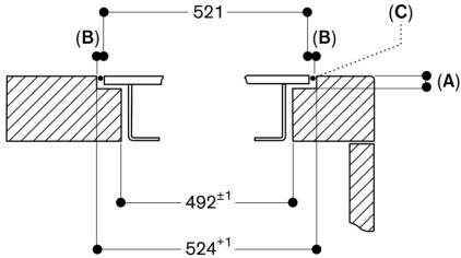
Sezione trasversale
