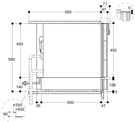
Vista laterale WS 461 sotto BS, BM, CM
