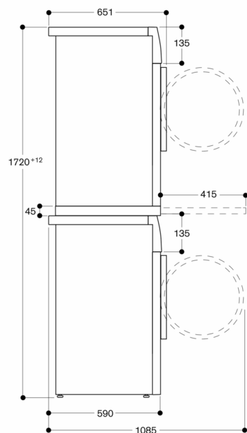
Vista laterale di WT 260 sopra WM 260 con accessorio kit di congiunzione
