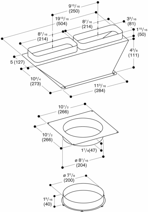
Dimensioni in pollici (mm)
