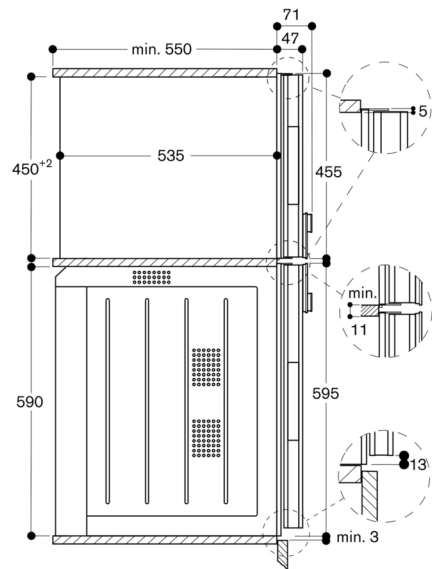
Vista laterale BM 454/455 su BO
