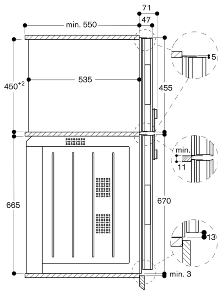
Vista laterale BM 484/485 su BO
