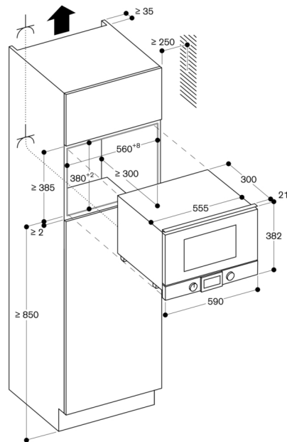
Montaggio in un mobile a colonna
