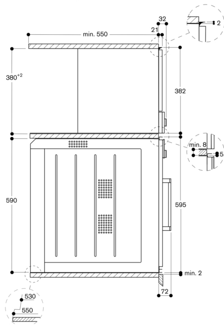
Vista laterale BMP 224/225 su BOP
