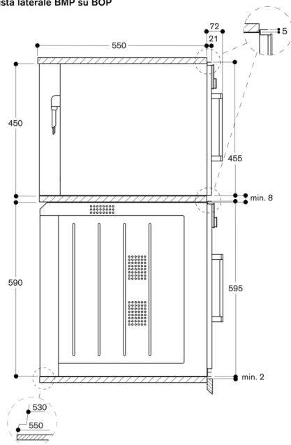
Vista laterale BMP su BOP
