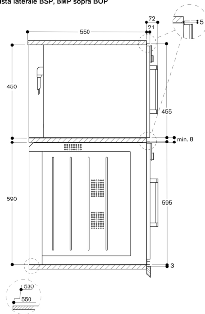
Vista laterale BSP, BMP sopra BOP
