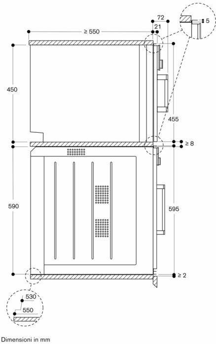
Vista laterale di BSP 220/250 su BOP
