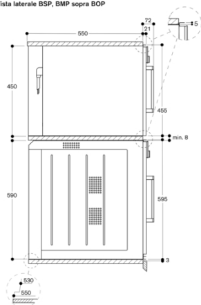
Vista laterale BSP, BMP sopra BOP
