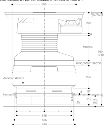
Vista frontale CV 28, con modulo a ricircolo CA 282 811
