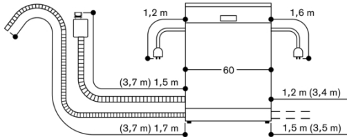
Dimensioni per il collegamento di una lavastoviglie larga 60 cm
