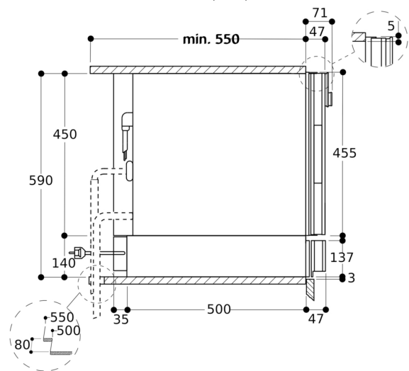
Vista laterale DV 461 sotto BS, BM, CM
