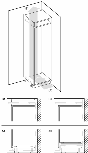
A: Ingresso aria ≥ 200 cm²; opzioni ventilazione A1 o A2 B: Uscita aria ≥ 200 cm²; opzioni ventilazione B1 o B2
