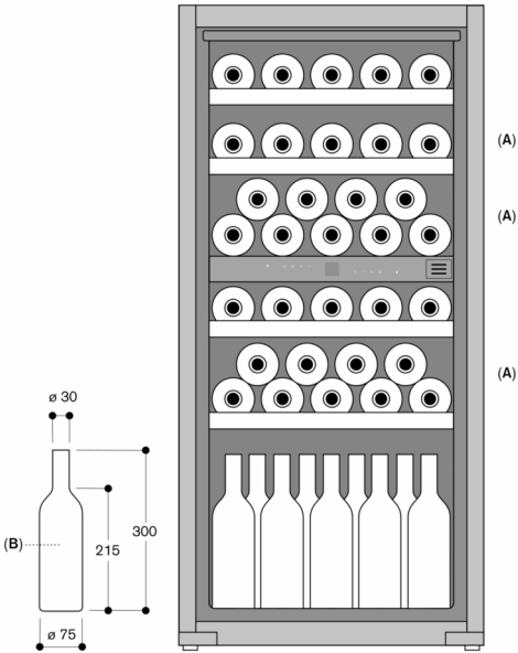
A: Area idonea allo stoccaggio di bottiglie magnum nella configurazione standard del vano B: 0,75 litri Dimensioni in mm
