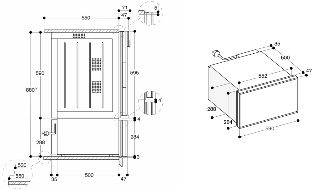
Vista laterale WS 462 sotto BO
