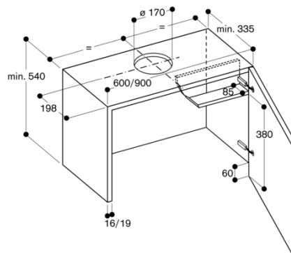
Bovenkast voor AF 210 met inbouwframe AA 210 460 / AA 210 490
