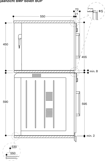
Zijaanzicht BMP boven BOP
