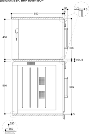
Zijaanzicht BSP, BMP boven BOP
