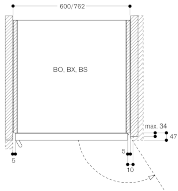
Ventilatiedoorsnede bij deurrand
