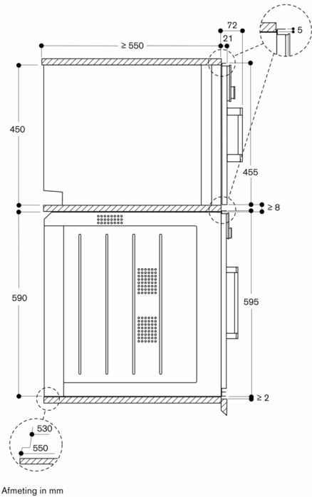
Zijaanzicht van BSP 220/250 boven BOP
