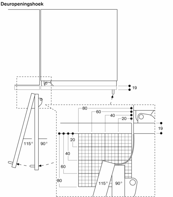
Deuropeningshoek De scharnierslag en de daaruit resulterende afstanden tot de naastliggende kasten en meubelgrepen kunnen afhankelijk van de plaatdikte in de tekening worden afgelezen. In de tekening is uitgegaan van een meubelfrontdikte van 19 mm.
