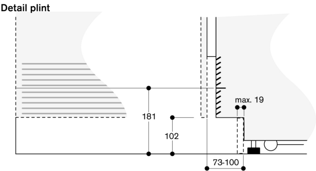
Detail plint Op basis van de standaard hoogte van het apparaat bedraagt de hoogte van de plint 102 mm. Maximale dikte van de plint 19 mm.
