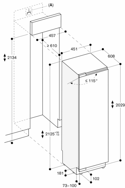
A: Stopcontact Maximale deurfrontmaten zijn gebaseerd op een speling van 3 mm Afmeting in mm
