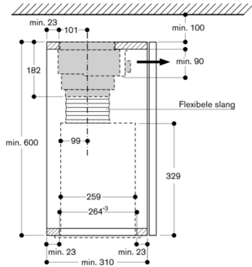
Dwarsdoorsnede bovenkast met AC 200 en AA 211 812
