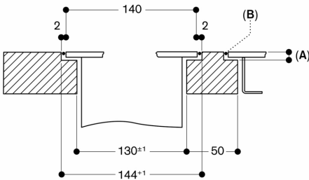
Dwarsdoorsnede
