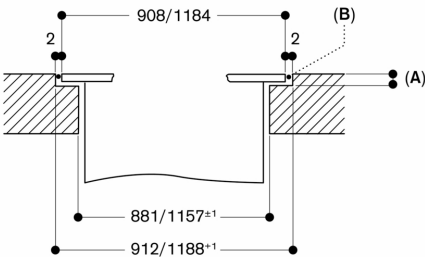
Longitudinale sectie
