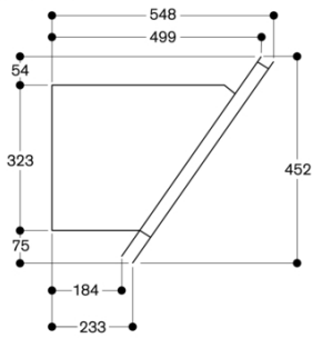
Zijaanzicht
