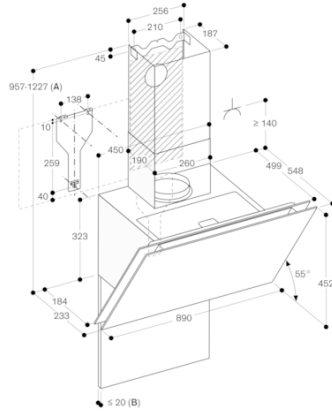
Luchtafvoer
