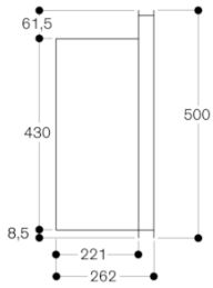
Zijaanzicht
