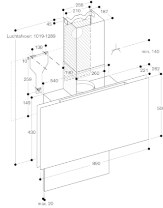
Luchtafvoer
