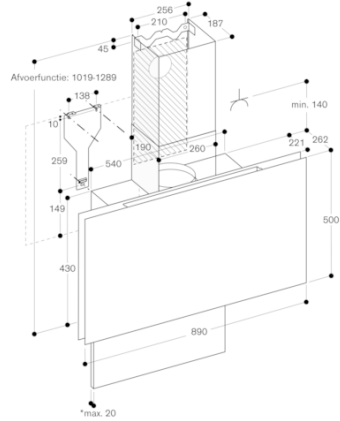
Afvoerfunctie
