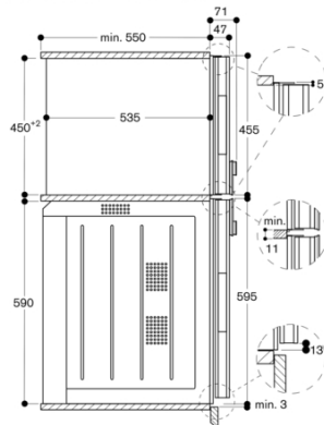
Zijaanzicht BM 454/455 boven BO
