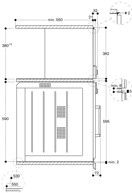
Zijaanzicht BMP 224/225 boven BOP
