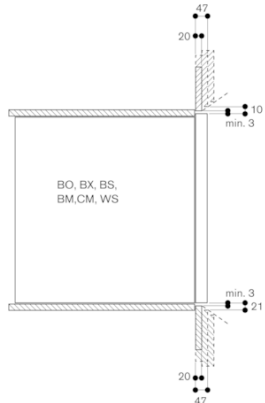
Luchtdwaarsnede aan de deurranden boven/onder
