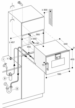
1 Stoptocontact Afmeting in mm
