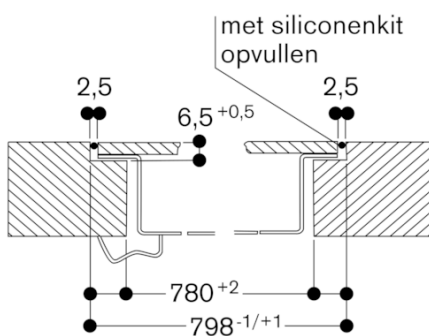
Langsdoorsnede
