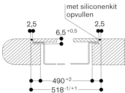
Dwarsdoorsnede
