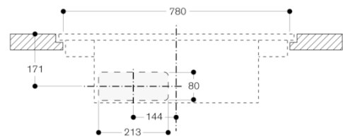
Voorbeeld - Meubeluitparing voor ongeleide circulatie - vlak (CA 082 010)
