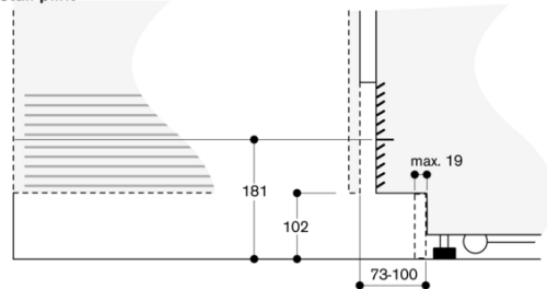
Detail plint
