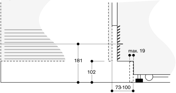
Detail plint
