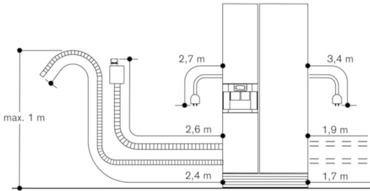
Aansluitmaten voor RX 496
