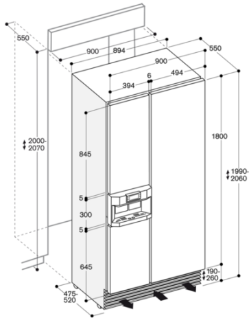
RX 496 200/290 Volledig integreerbaar
