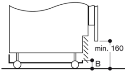
Zijaanzicht sokkelzone
