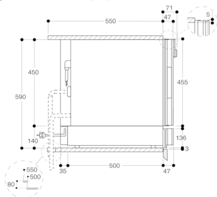
Zijaanzicht WS 461 onder BS, BM, CM
