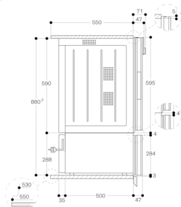
Zijaanzicht WS 462 onder BO
