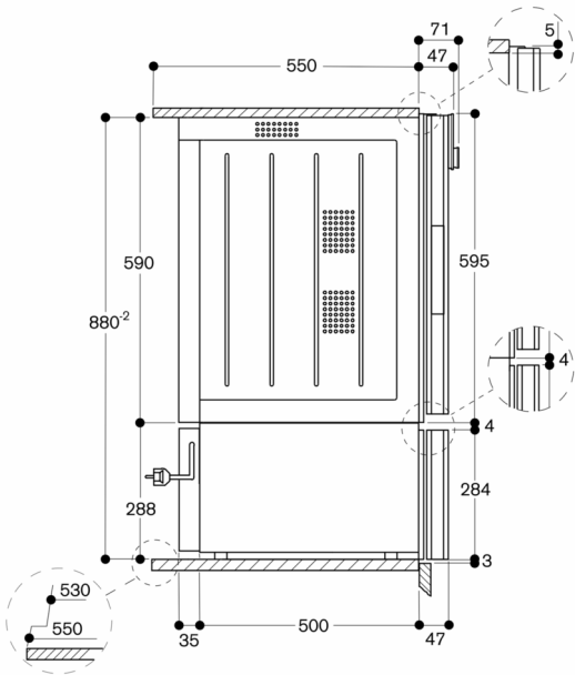
Zijaanzicht WS 462 onder BO
