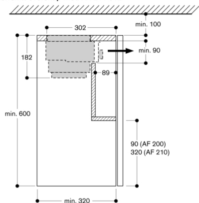
Tverrsnitt overskap med AA 211 812
