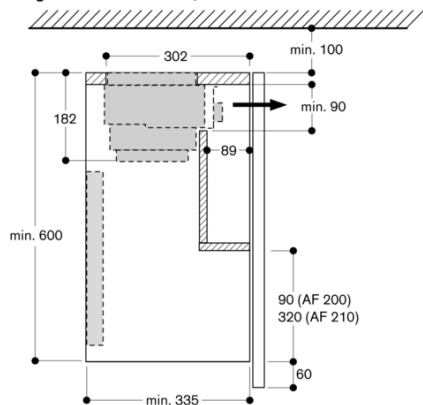
Tverrsnitt overskap med AA 211 812 og senkingsramme AA 210 490/460
