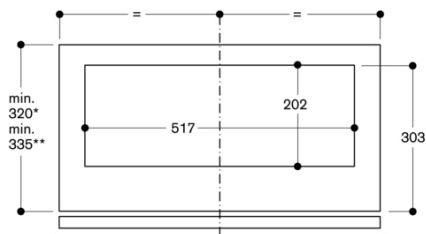
Visning ovenfra overskap med AA 211 812
