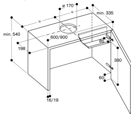
Overskap til AF 210 med senkingsramme AA 210 460 / AA 210 490
