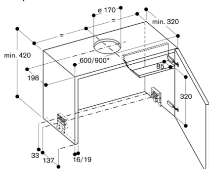
Overskap til AF 210
