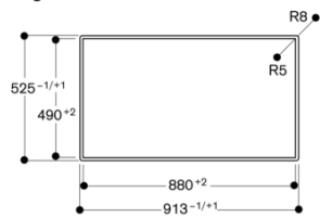
Visning ovenfra
