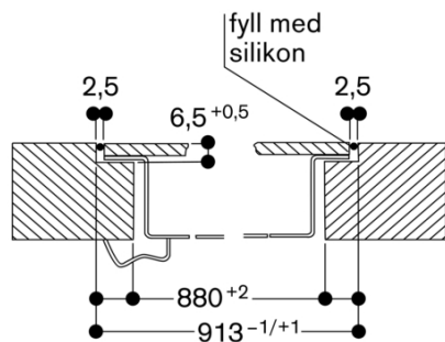
Lengdesnitt
