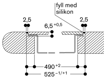
Tverrsnitt
