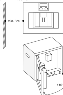
Hjørneinnbygging venstre
