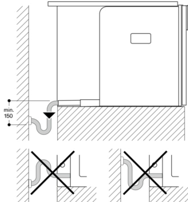
Avløpstilkobling
