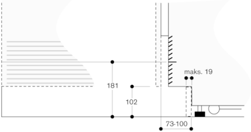
Detalj sokkel
