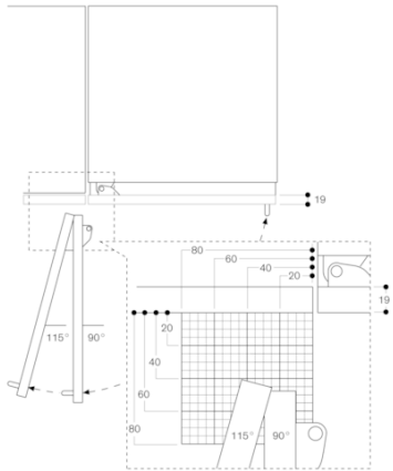
Døråpningsvinkel
