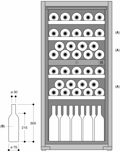
A: Egnet område for lagring av magnumflasker i standardkonfigurasjon B: 0,75 liter Mål i mm
