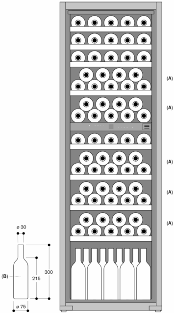
A: Egnet område for lagring av magnumflasker i standardkonfigurasjon B: 0,75 liter Mål i mm
