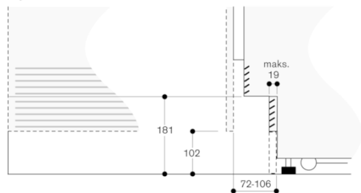
Detalj sokkel
