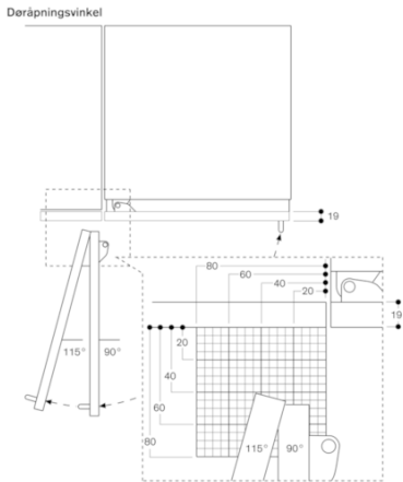
Hvor stor plass hengselet krever, og hvilke avstander til tilstøtende kjøkkenelementer og håndtak dette resulterer i, kan leses av på tegningen (men avhenger av fronttykkelsen). Tegningen tar utgangspunkt i en elementfront som er 19 mm tykk.
