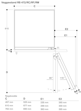
På tegningen er det tatt utgangspunkt i en møbelfronttykkelse på 19 mm og en høyde på Gaggenau møbelhåndtak på 49 mm.
