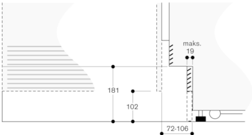
Med utgangspunkt i apparatets standardhøyde er høyden til sokkellisten 102 mm. Maks. tykkelse til sokkellisten er 19 mm.
