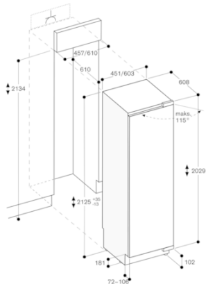
De maksimale derfrontmålene er dimensjonert for spaltmål på 3 mm.
