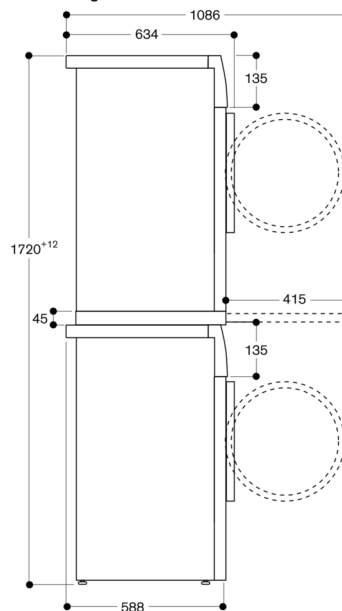
WT 260 over WM 260 sett fra siden med monteringssett WA 032 001
