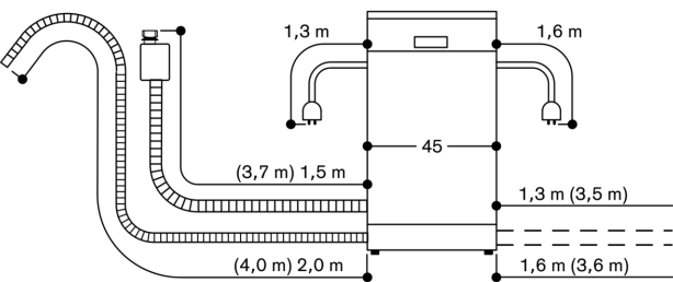
Wymiary przyłączeniowe do zmywarek o szerokości 45 cm
