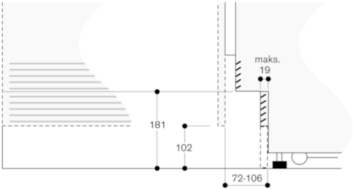
Rysunek szczegółowy cokołu
