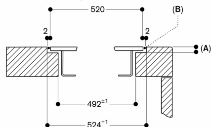
Przekrój poprzeczny
